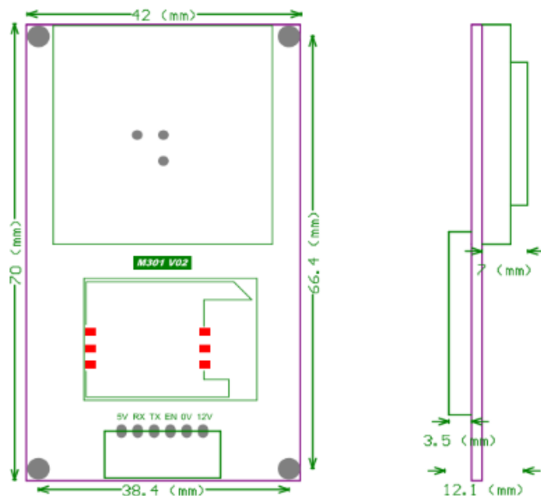
M301尺寸图(mm)
